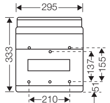
Quadros de distribuição KV 12 módulos
