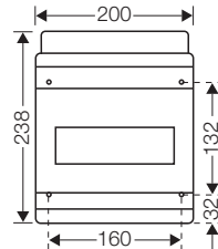
Quadros de distribuição KV 3 x 12 módulos
