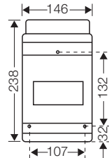
Quadros de distribuição KV 6 módulos
