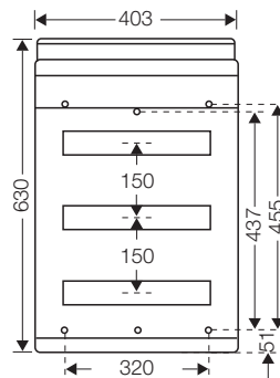
Quadros de distribuição KV 3 x 18 módulos
