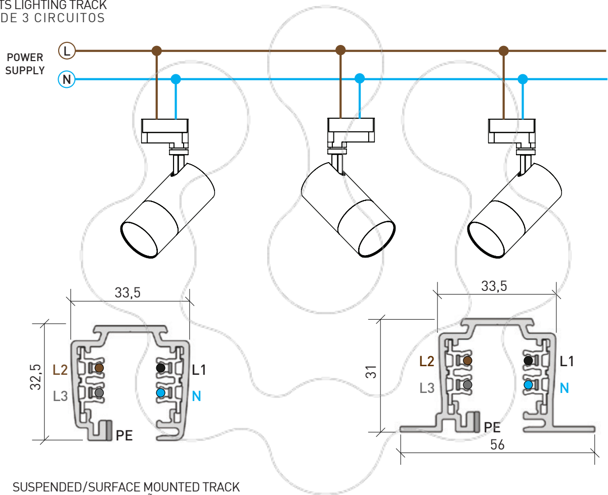
RECESSED TRACK . CALHA DE ENCASTRAR
