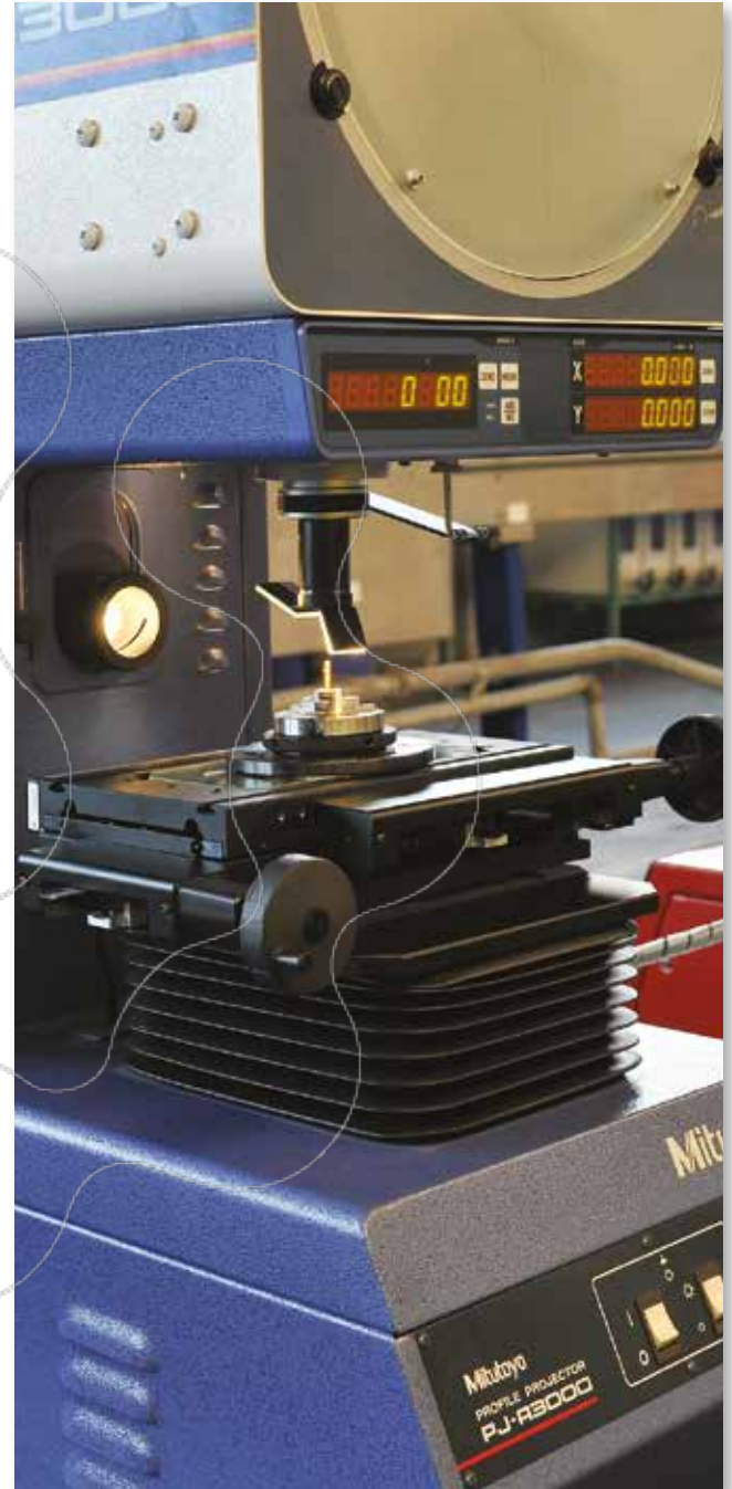
Profil projektör ile geometrik ölçümler yapılır.
