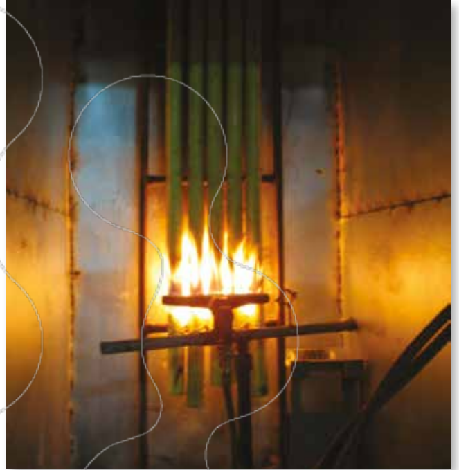
Demetlenmiş kabloların yanması testindeki bir kablo numunesi.
