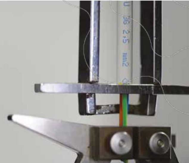
Sıyırma testi altındaki bir numune.
