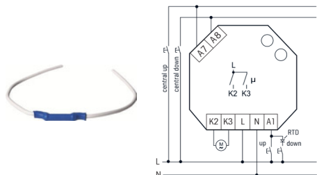
Esquema de ligação com EGS61Z230
