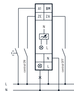
Esquema de ligação
