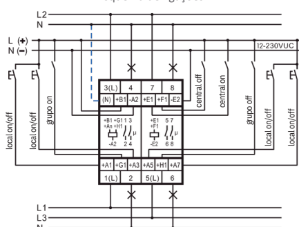
Esquema de ligações
